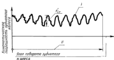
I — кривая кинематической погрешности зубчатого колеса; II — один оборот зубчатого колеса
